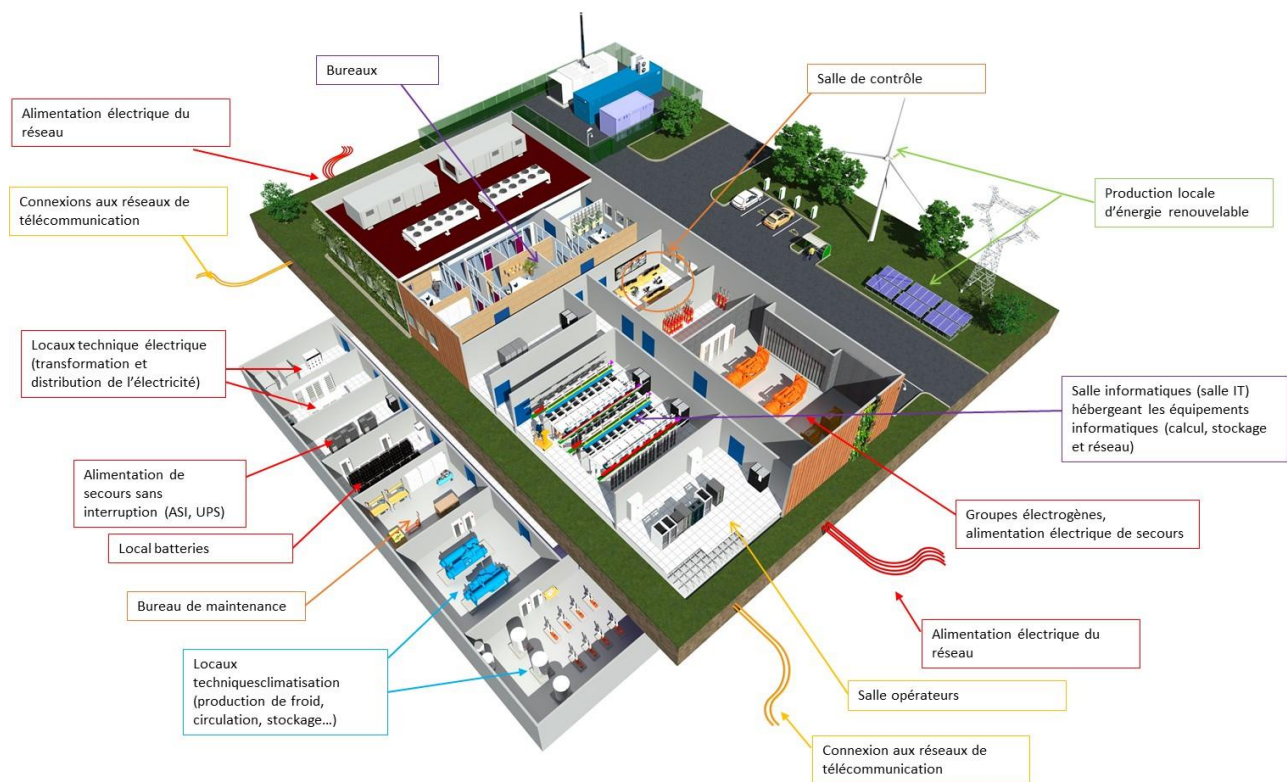
Figure 1 - Représentation d'un datacenter - Source APL DATA CENTER
