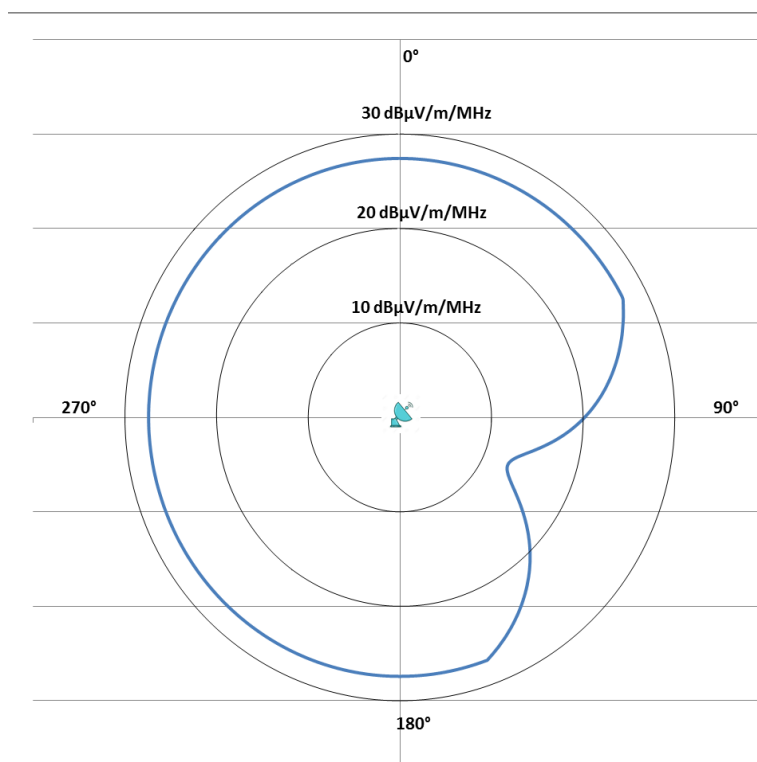
Figure 7 : Limite de champ en direction du site de Toulouse-3 au-dessus de 3840 MHz
