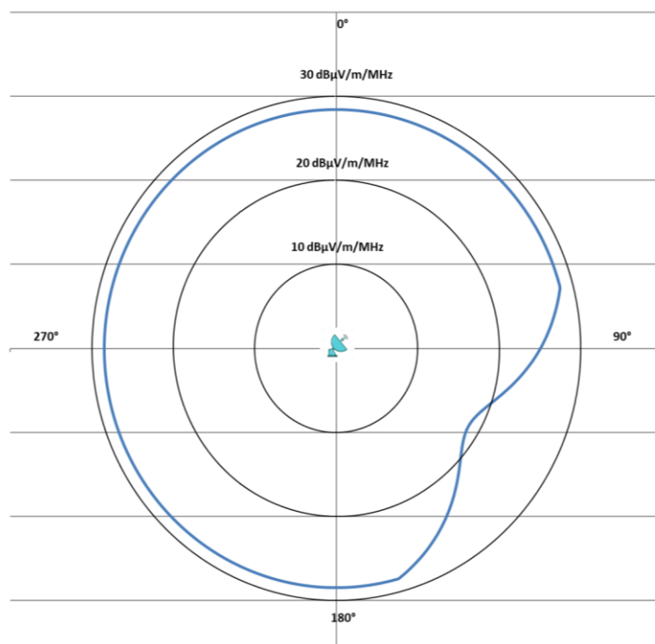
Figure 19 : Limite de champ recommandée en direction du site de Fréjus entre 3814 et 3823 MHz
