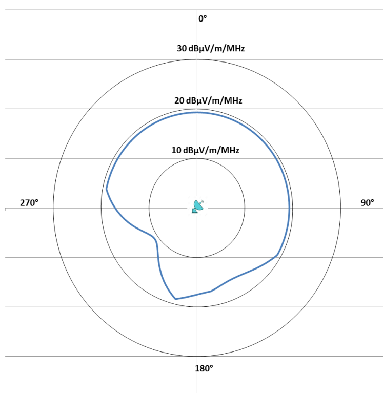
Figure 5 : Limite de champ en direction du site de Toulouse-1, au-dessus de 3840 MHz
