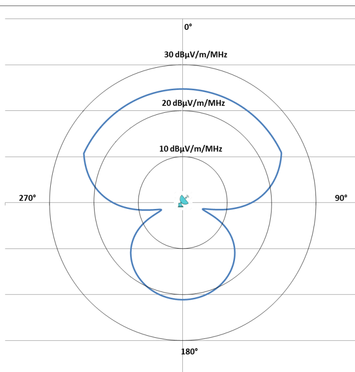
Figure 12 : Limite de champ en direction du site de Rambouillet au-dessus de 3840 MHz
