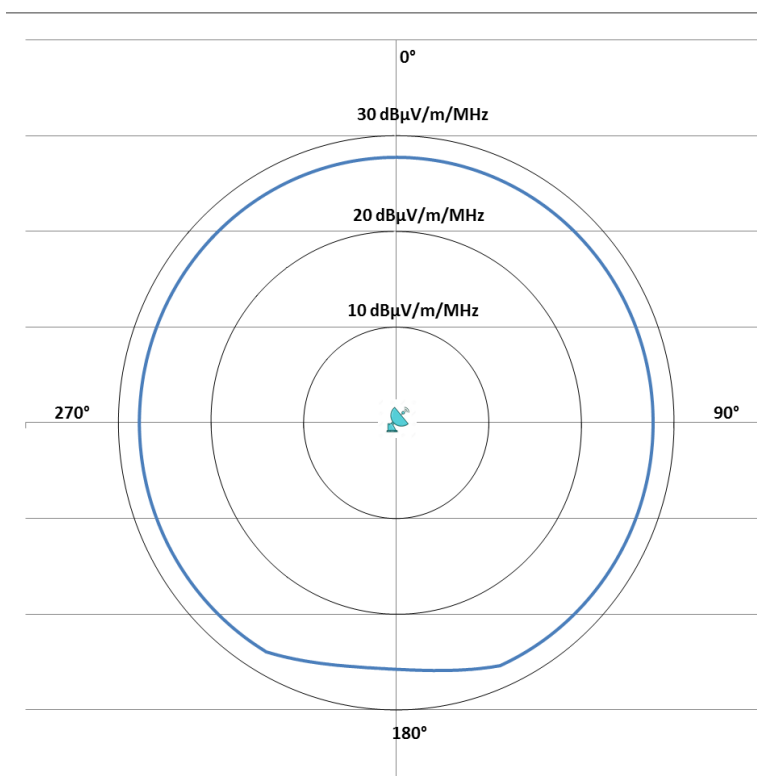
Figure 6 : Limite de champ en direction du site de Toulouse-2 au-dessus de 3840 MHz
