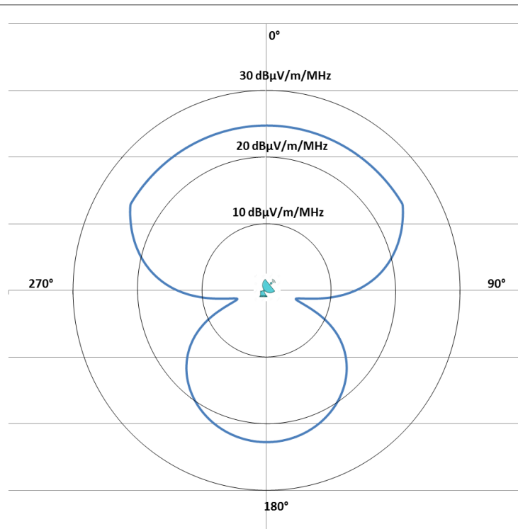
Figure 16 : Limite de champ en direction du site e Fréjus au-dessus de 3840 MHz
