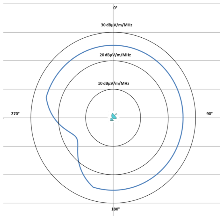
Figure 17 : Limite de champ en direction du site de Fréjus entre 3800 et 3833 MHz et entre 3837,4 et 3838,4 MHz
