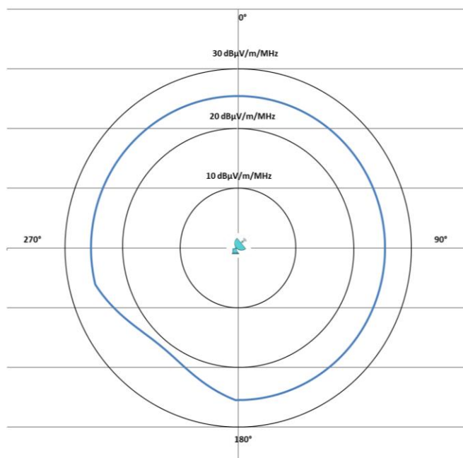
Figure 18 : Limite de champ en direction du site de Fréjus entre 3804,4 et 3838 MHz
