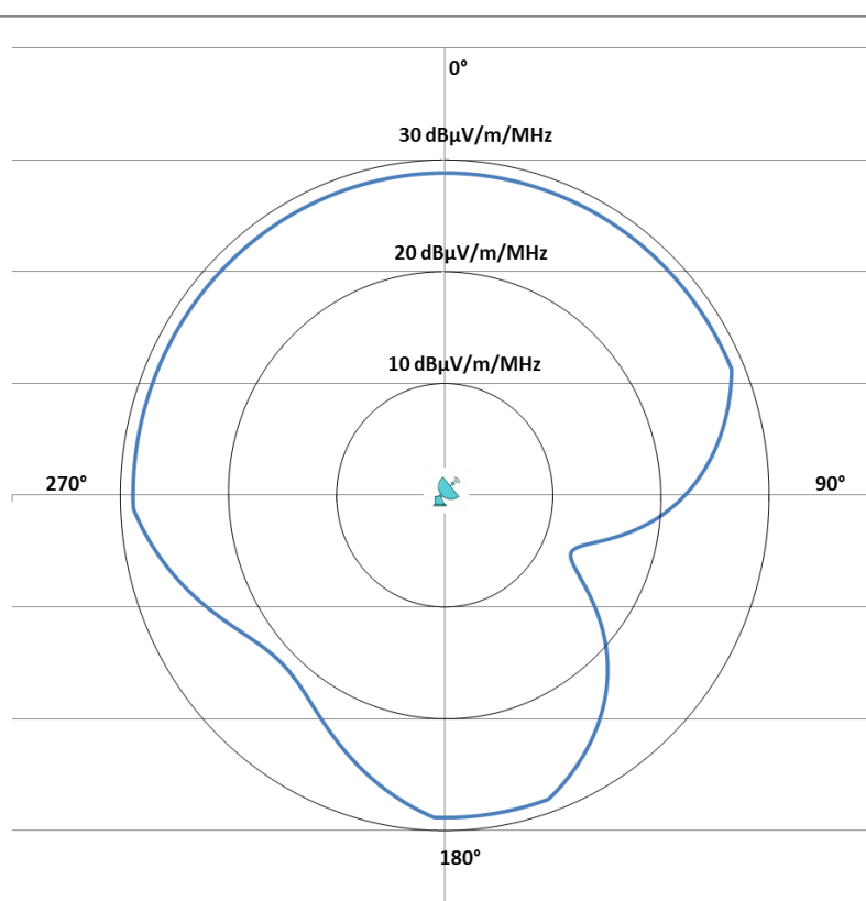
Figure 4 : Limite de champ en direction du site de Chevilly-Larue au-dessus de 3840 MHz
